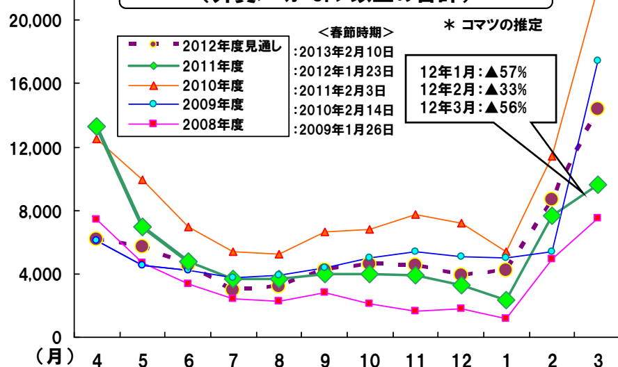
油圧ショベルの月別需要推移 (外資メカ: 6トン以上の合計)
