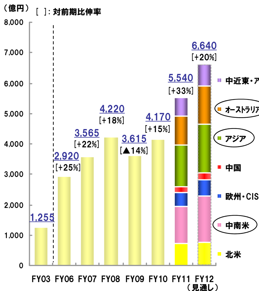
鉱山機械 地域別売上高(部品・サービス含む)
