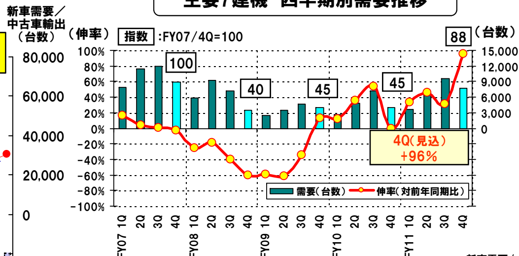
油圧ショベルのストック台数、新車需要・中古車輸出台数推移
